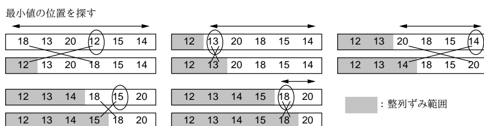
図 3: 単純選択法
