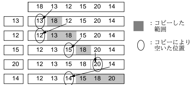
図 4: 単純挿入法
