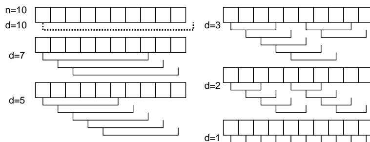
図 6: コムソート
